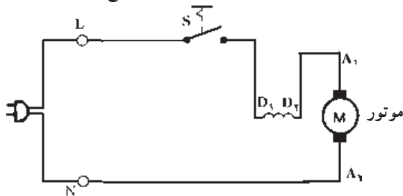
شکل ۳-۵۱- مدار الکتریکی چرخ گوشت‌های معمولی و بدون معکوس‌کننده‌ی دور موتور
